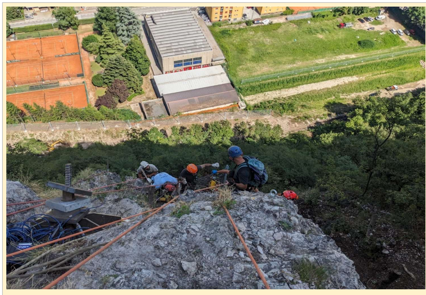
Verifica tiranti in parete (foto I. Vigna)
